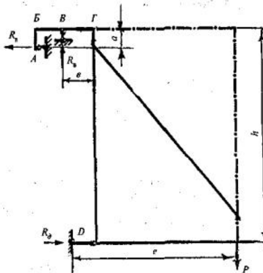
Рисунок 6 - Расчетная схема навесных лесов
