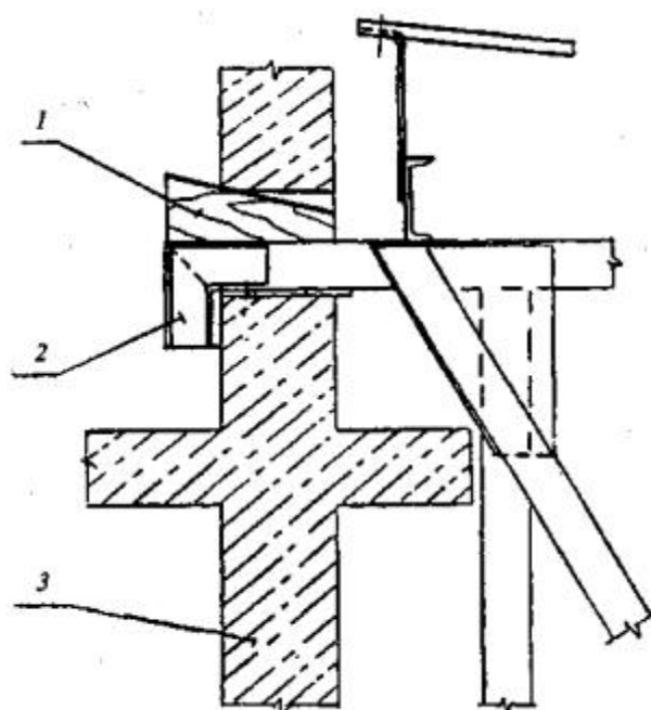
1- клин деревянный; 2- кронштейн лесов; 3- стена.
