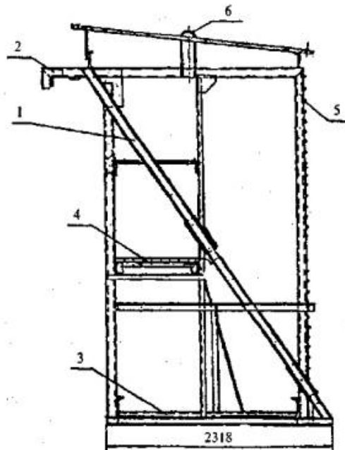
Рисунок 2 - Одноярусные леса
