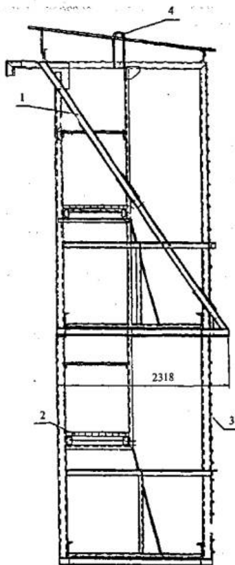
Рисунок 2 - Одноярусные леса
